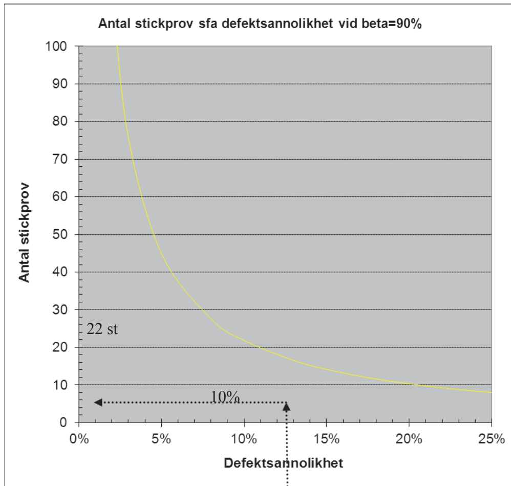
Antal stickprov som funktion av defektsannolikhet vid \beta=90\%
