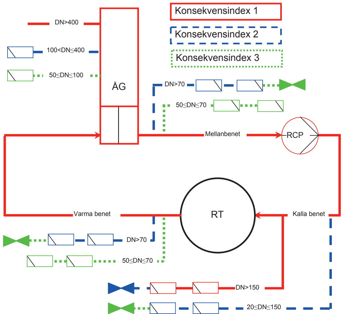
Schematisk bild över konsekvensindex för rörledningar och tryckbärande anordningar i PWR
